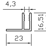
No: 36917 F Profili 23x16,5
