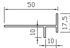
No: Y41047 Damlalık Profili
