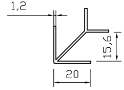
No: 10127 Köşe Profili max 11mm seramik
